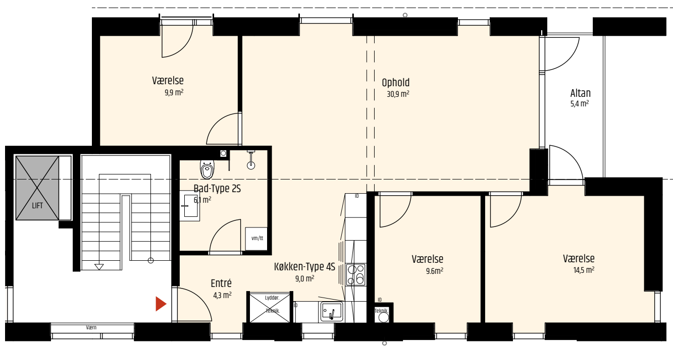
Type F 1:100
