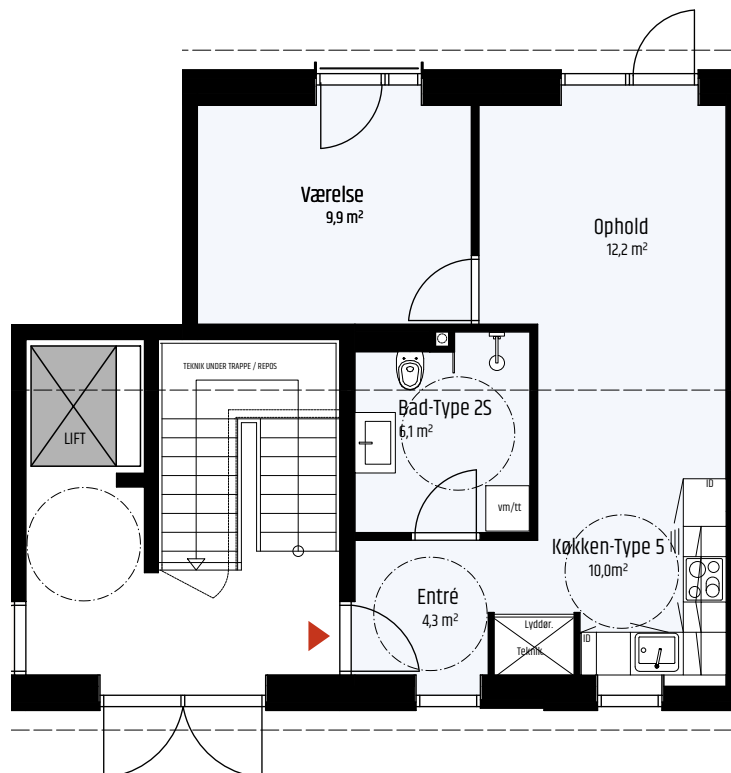
Type I 1:100
