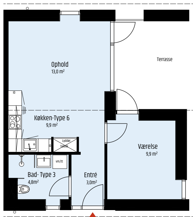
Type H 1:100
